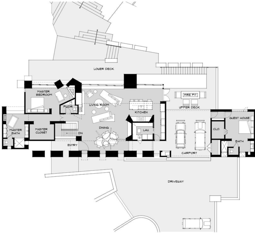
3900 RONDA RD - PEBBLE BEACH UPPER FLOOR PLAN
